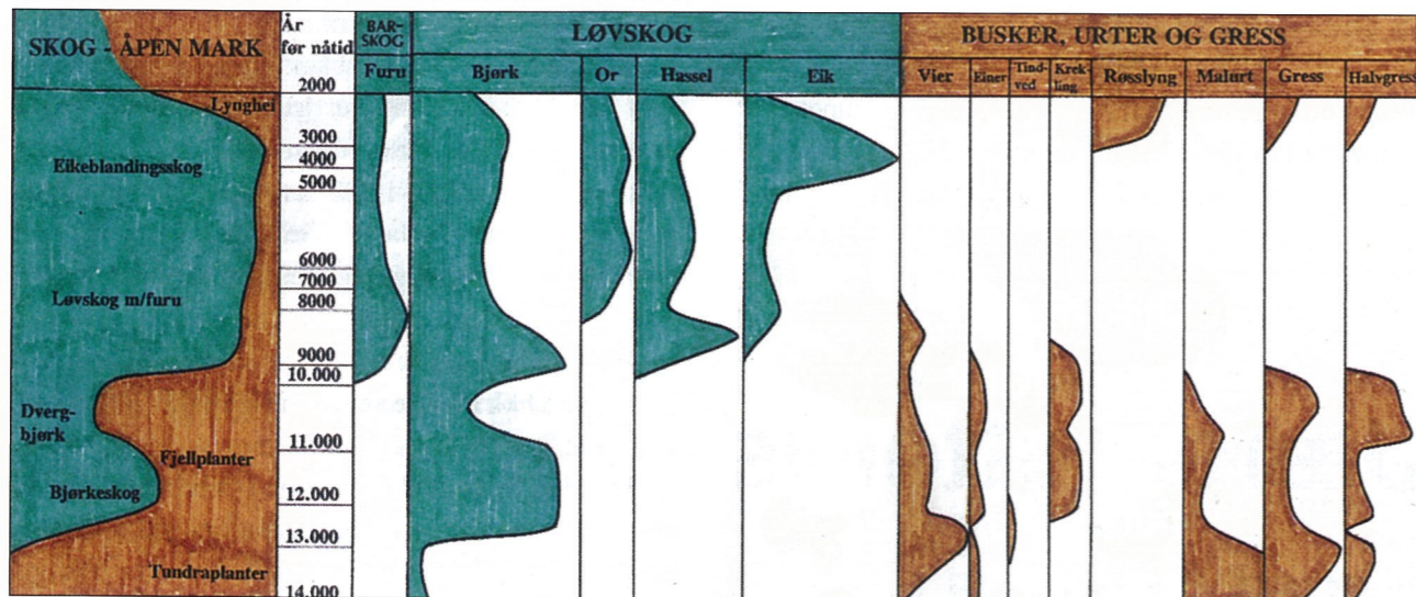
Pollendiagram som viser hovedtrekkene i vegetasjonsutviklingen på Jæren etter istiden. Når en leser diagrammet vannrett kan man se hovedelementene i plantedekket til forskjellige tider. Når en leser diagrammet nedenfra og oppover, kan man følge vegetasjonsutviklingen over tid. Pollendiagrammet er en forenklet og sammensatt utgave av K. Fægri's diagrammer fra Alvevatn (1935) og Egebakken (1989).
