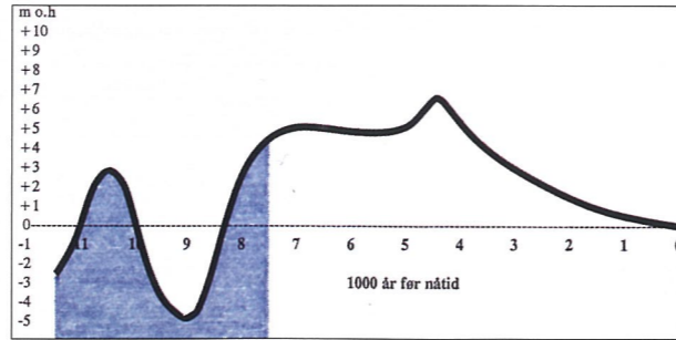
Strandforskyvingskurve for Sør-Jæren for hele perioden etter istiden. Strandens posisjon rundt Hå-elva har flyttet opp og ned nærmest som en jojo. Kurven illustrer hvor høyt i landskapet vanlig høyvann nådde til forskjellige tider.
