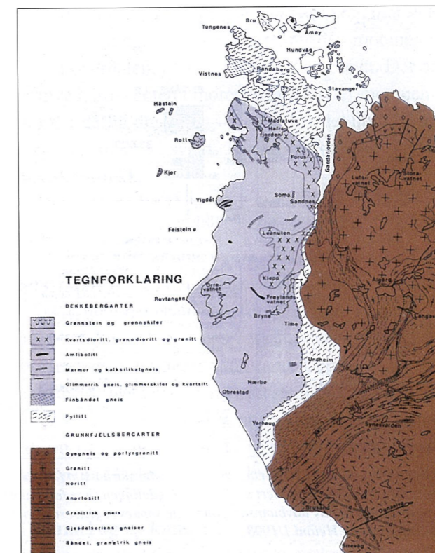
Geologisk kart over Jæren. Fra Lye et al 1979, modifisert av Thomsen 1988. "Frå Haug & Heidni" 3/1999.
