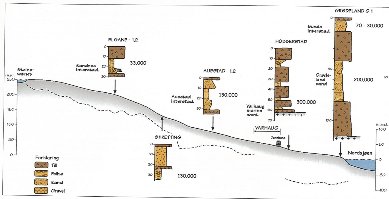
Figuren viser en profil fra Steinsvatnet, gjennom Varhaug og ut mot havet. Den stiplede linjen viser dyp til fjell i henhold til seismiske undersøkelser. Det er plassert søyler over lagdelingen (noe forenklet) funnet i boringene som ble utført i området i årene 1993 til 1995. Navn og alder på en del av havbunnsavsetningene som er registrert er vist. Kjelde: Haug og Heidni 1/1998.
